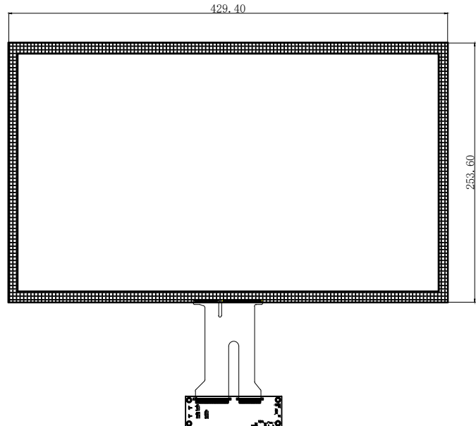
背视图
