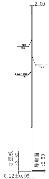
侧视图
