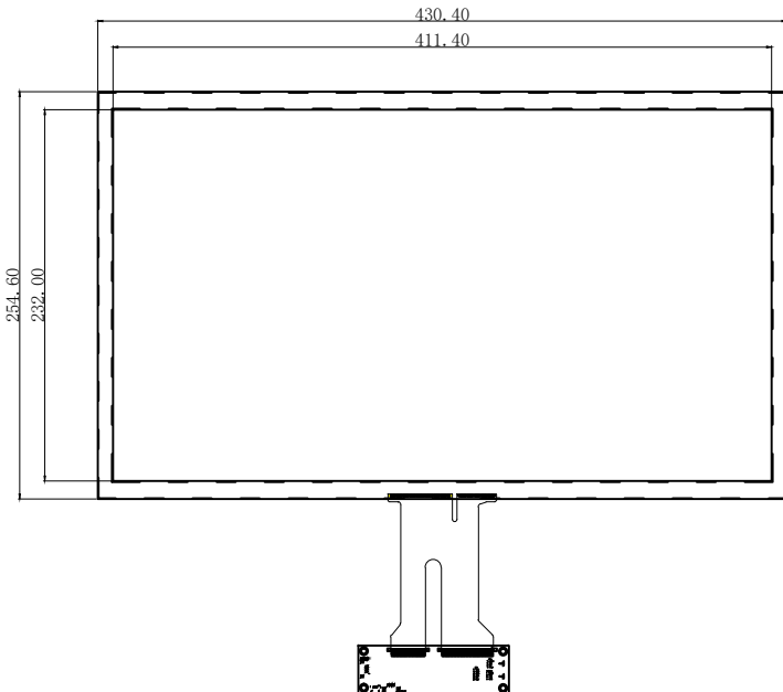
正视图
